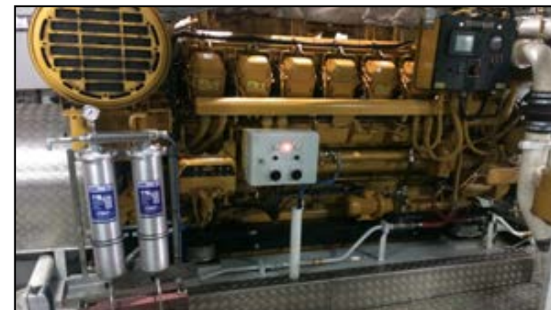
AL600 Doppelsystem für Öl an einem Generator. AL600 double system for oil on a generator.
