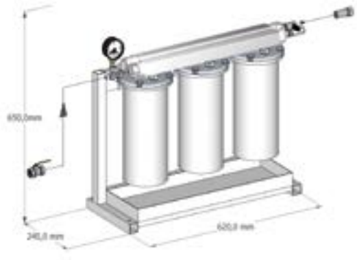
Trippelsystem AL300 für Öl mit Manometer Triple system AL300 for oil with pressure gauge
