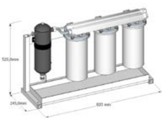
Trippelsystem AL300 für Diesel mit Wasserseparator WS800 Triple system AL300 for diesel with water separator WS800
